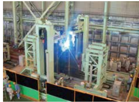
セパレート型ツイン溶接ロボット Separate type twin welding robot
